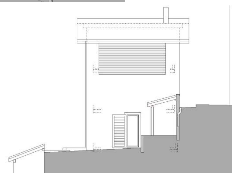
Süd- und Westfassade
