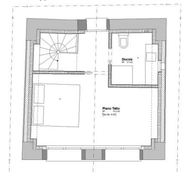
Grundrisse 1. und 2. Obergeschoss
