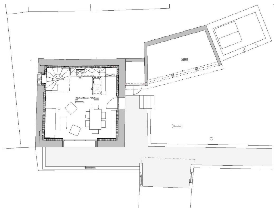
Grundriss Erdgeschoss mit Umgebung
