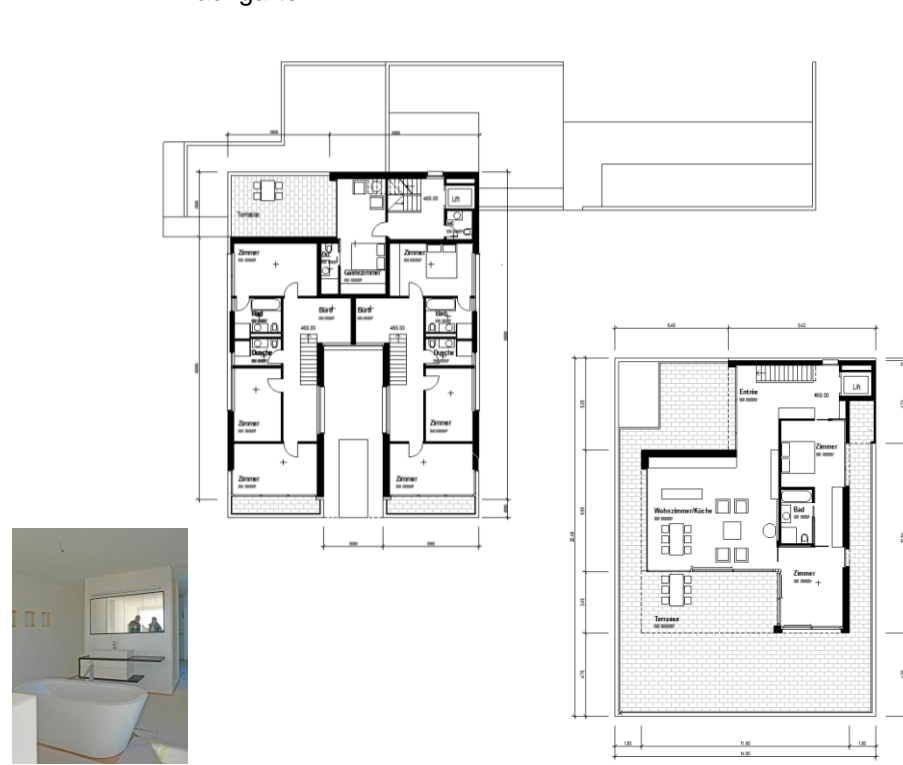
Grundriss Obergeschoss und Attika
