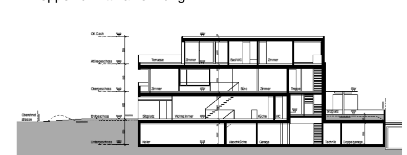
Treppe zur Attikawohnung
