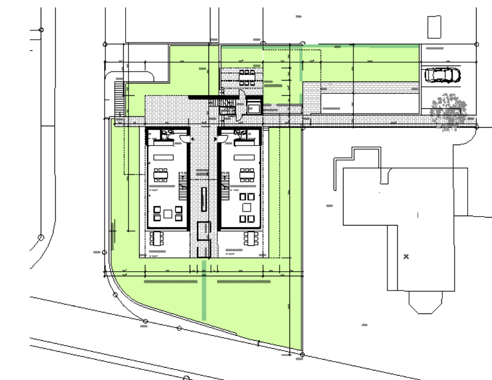
Grundrisse Erdgeschoss mit Umgebung
