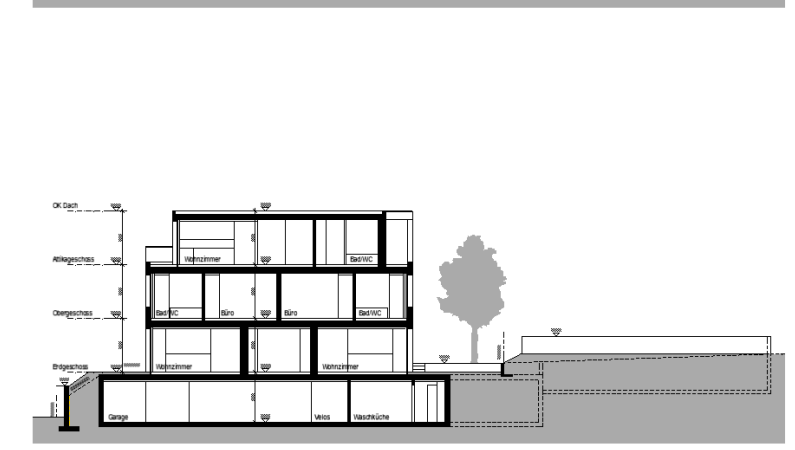
Längsschnitt und Querschnitt
